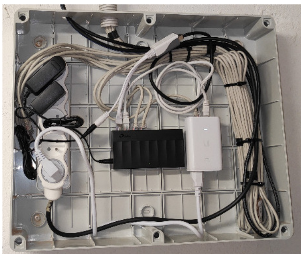
Rozvaděč k UNIFI wifi v Sokolovně.
